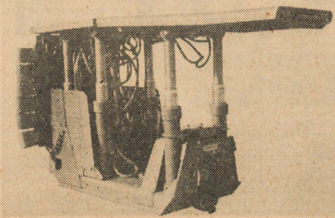
DOWTY — 6-cio stojakowa sekcja o podporności 240 t i zastosowana w ścianie 1 a pokład 415/I-3
