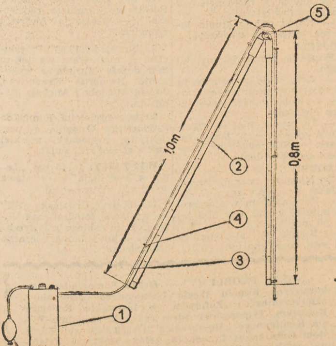
Schemat sondy do wykrywania metanu OBJAŚNIENIE: 1 — metanometr, 2 — drążek z drewna, 3 — wężyk gumowy, 4 — uchwyt na wężyk, 5 — przegub usztywniony śrubą z motylkową nakrętką
